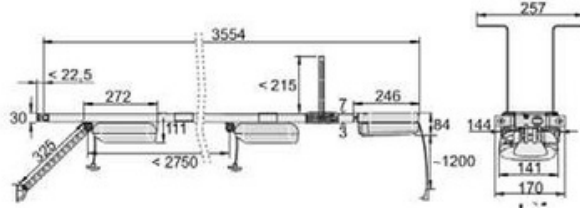
SOMMER base+ schéma s rozmermi (v mm)
